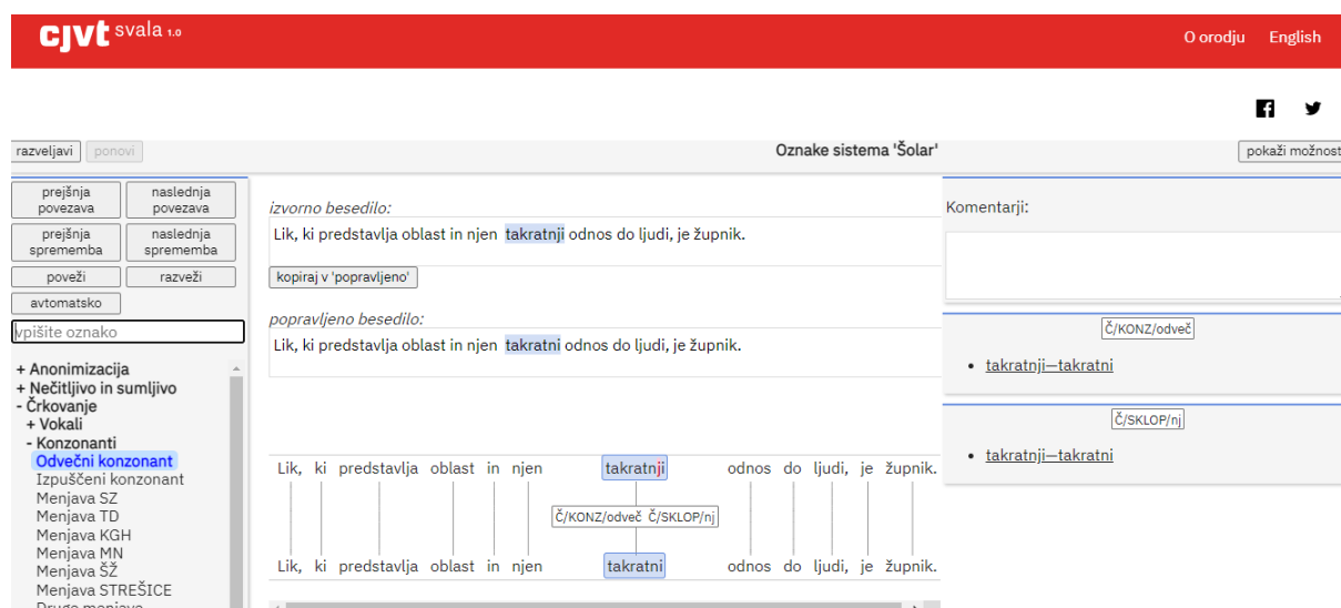
Slika 8: Primer izvirnega in popavljenega besedila v vmesniku CJVT-Svala s sistemom oznak za Šolar
